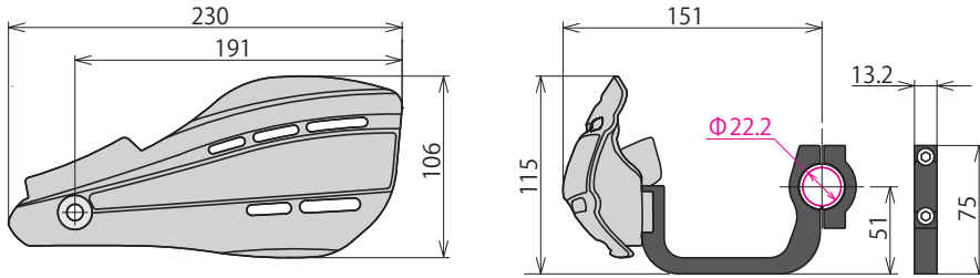
寸法図 (mm)
