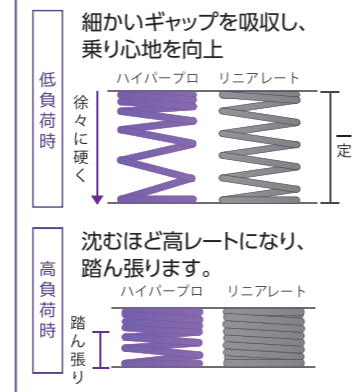
(フロントスプリング+リアスプリング)
