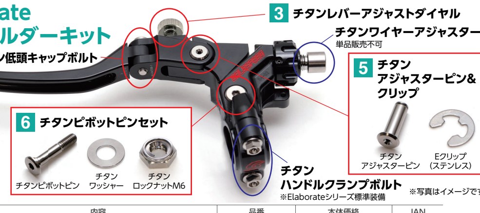
チタン ハンドルクランプボルト ※Elaborateシリーズ標準装備
