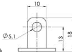
L字ステー寸法
