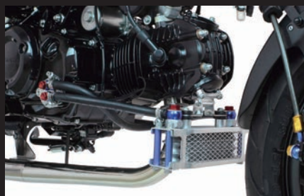
装着写真 (07-07-0421)
