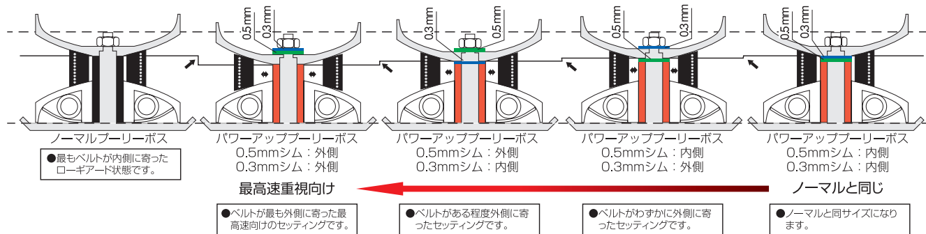
シムの組み合わせでブリーボスの長さを変える事で加速特性のセッティングが可能です。
