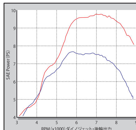
テスト車両:CT125 (JA55) ■ハイパーチューニングキット+スポーツマフラー ■ノーマルエンジン+ノーマルマフラー
