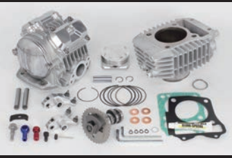
スーパーヘッド4V+R ポアアップキット181cc (シルバー仕様) (01-05-0173)
