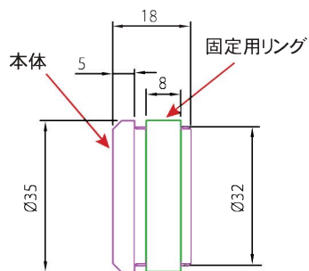
エアーインテークキット概略図
