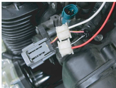
配線の接続先は、インジェクターカブラーハーネスとシリンダーヘッドボルト
