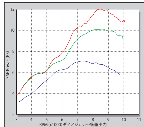
テスト車両:スーパーカブ110(JA07) ハイパーSステージボアアップキット125cc(FIコン付属) +ボンバーマフラー ■ビッグスロットルボディ仕様 ■ノーマルスロットルボディ仕様 ■ノーマルエンジン+ノーマルマフラー
