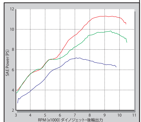
テスト車両:スーパーカブ110 ハイパーSステージボアアップキット125cc(FIコン2付属) +ボンバーマフラー ■ビッグスロットルボディ仕様 ■ノーマルスロットルボディ仕様 ■ノーマルエンジン+ノーマルマフラー
