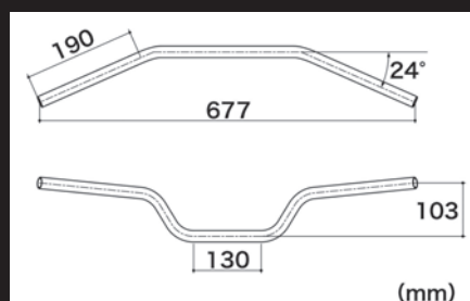
寸法図
