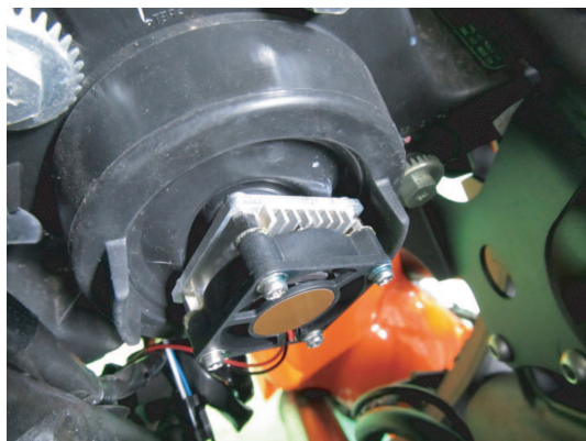
LEDバルブキット標準のファンの取付け状態
