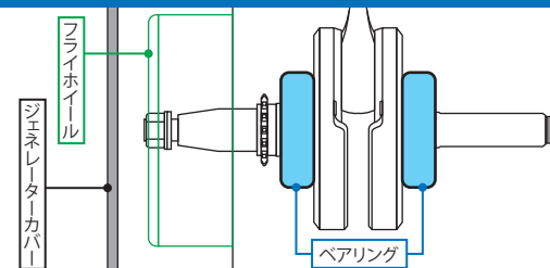
■クランクシャフトサポートアダプター装着イメージ図 3点支持
